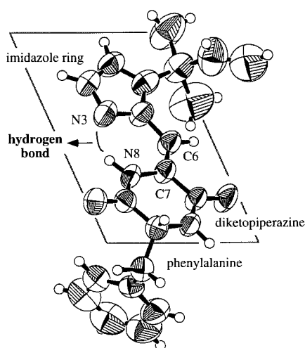
Figure 2. Crystal structure of (+)-phenylahistin (ORTEP).
